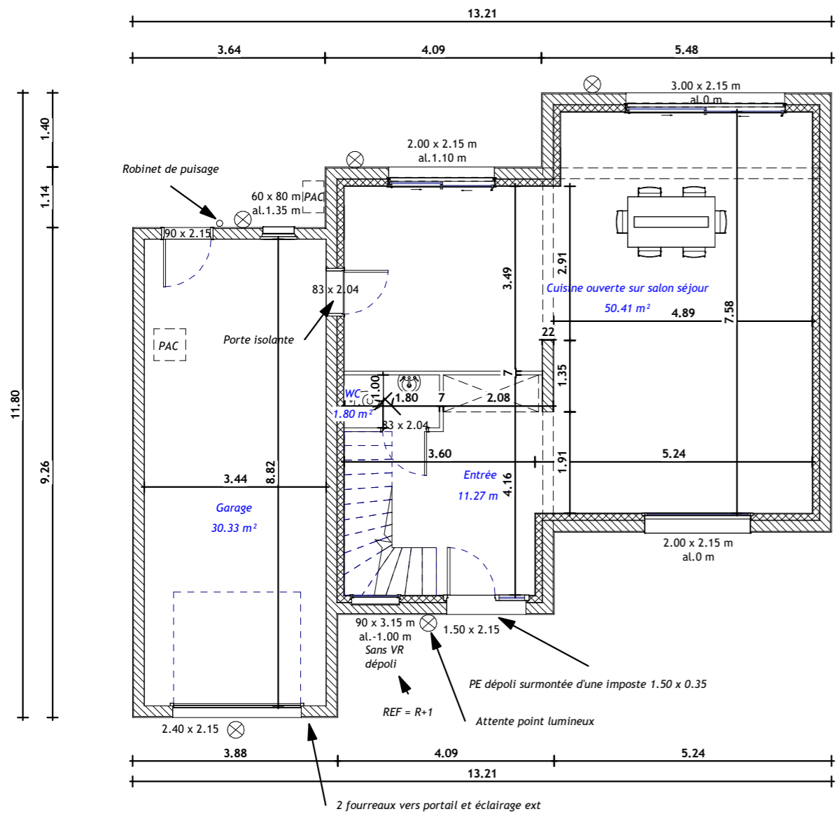
2 RDC Ech : 1 : 100
