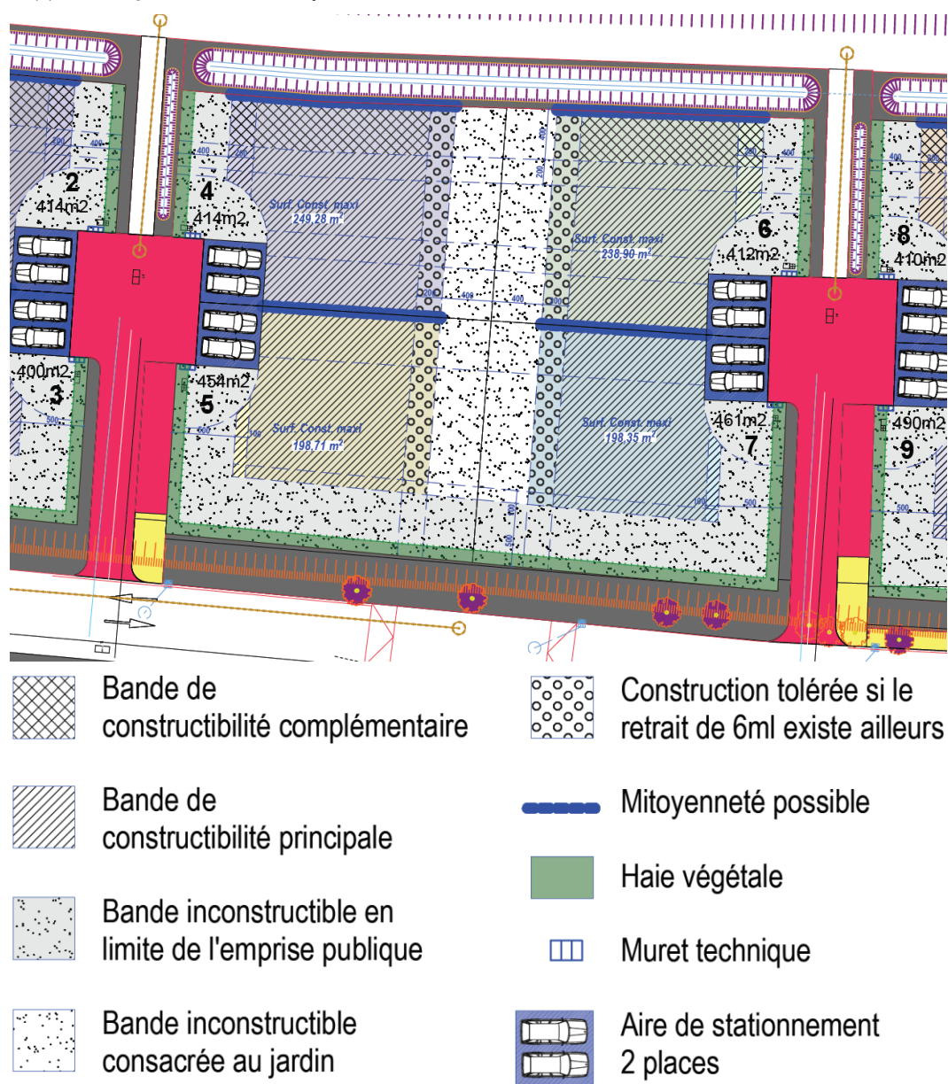
Figure 2 : Exemple de schéma d'implantation type d'une fiche de lot avec limite mitoyenne imposée
