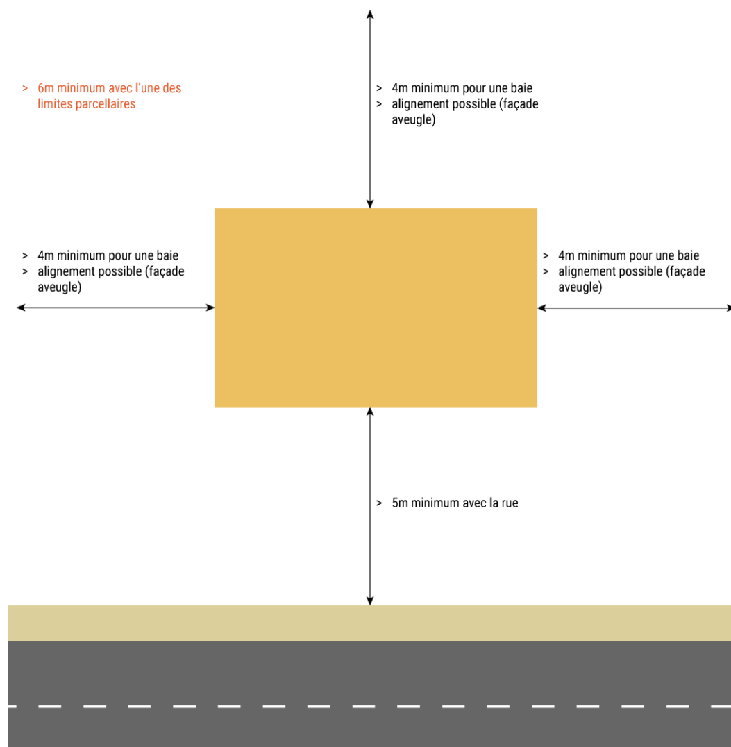
Figure 1 : cas général d'implantation de la construction principale
